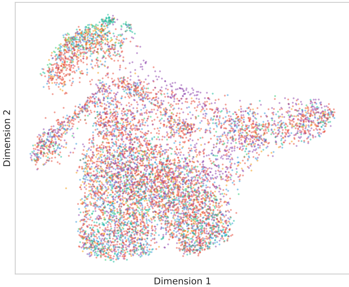
Geneformer - UMAP
