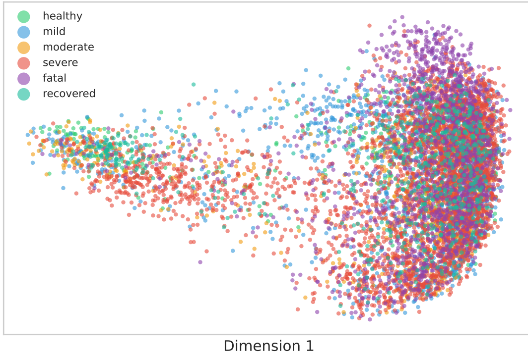
PCA (Var: 20.2%, 15.5%)
