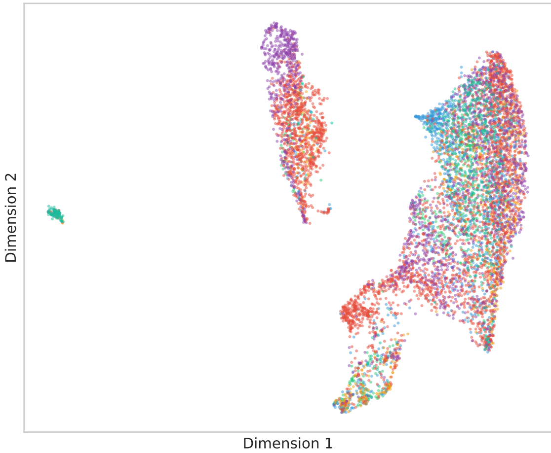
UCE - UMAP
