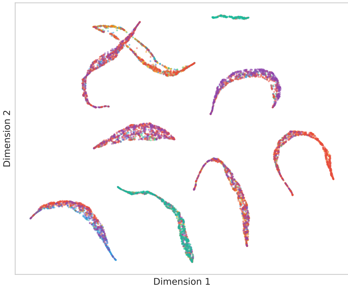
scGPT - UMAP
