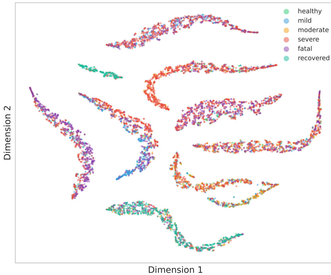
scGPT - tSNE
