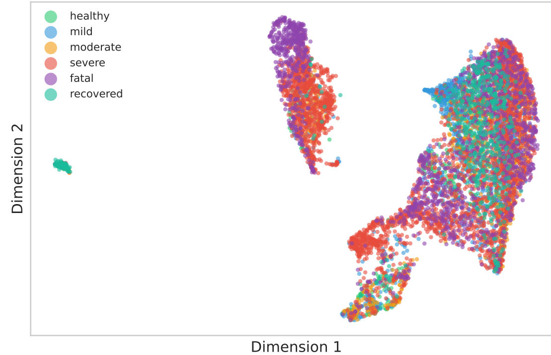
UMAP
