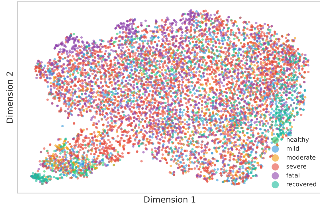
t-SNE
