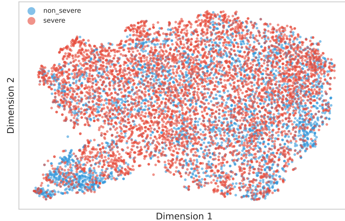
t-SNE
