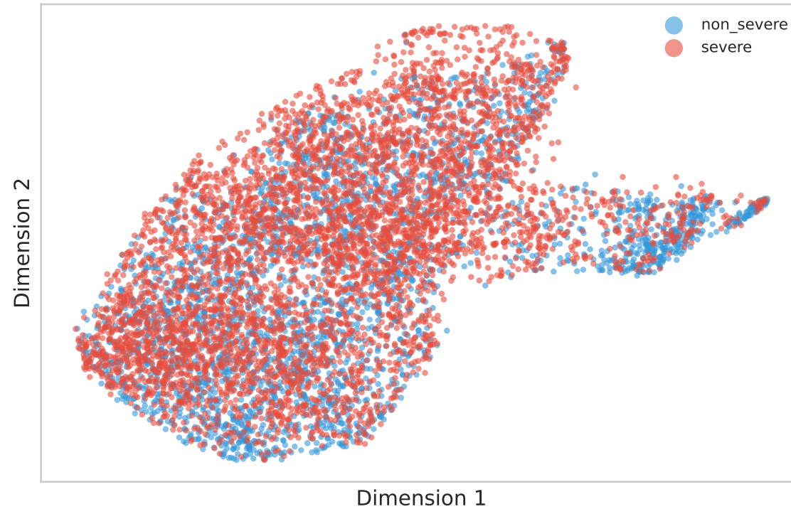
UMAP
