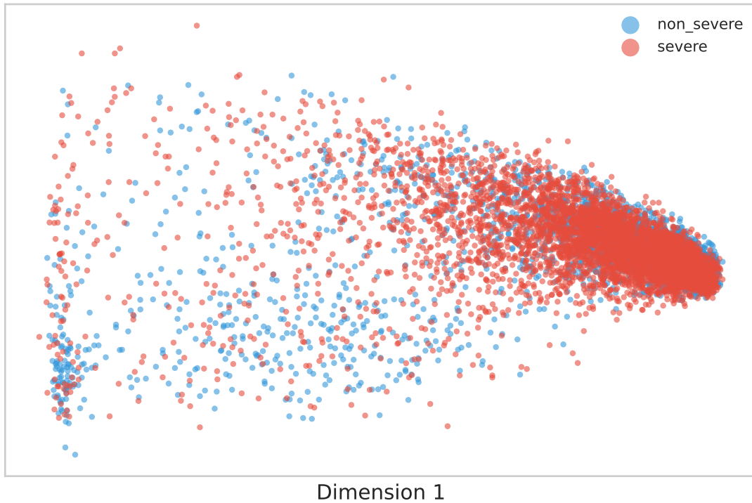
PCA (Var: 55.3%, 5.7%)
