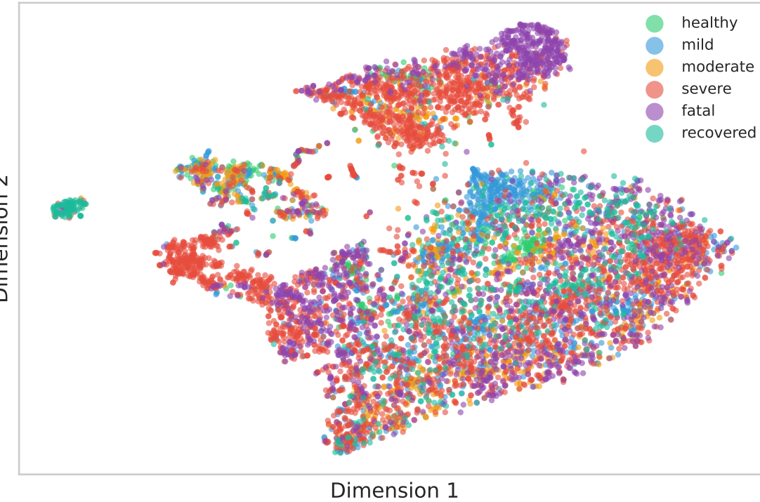
t-SNE
