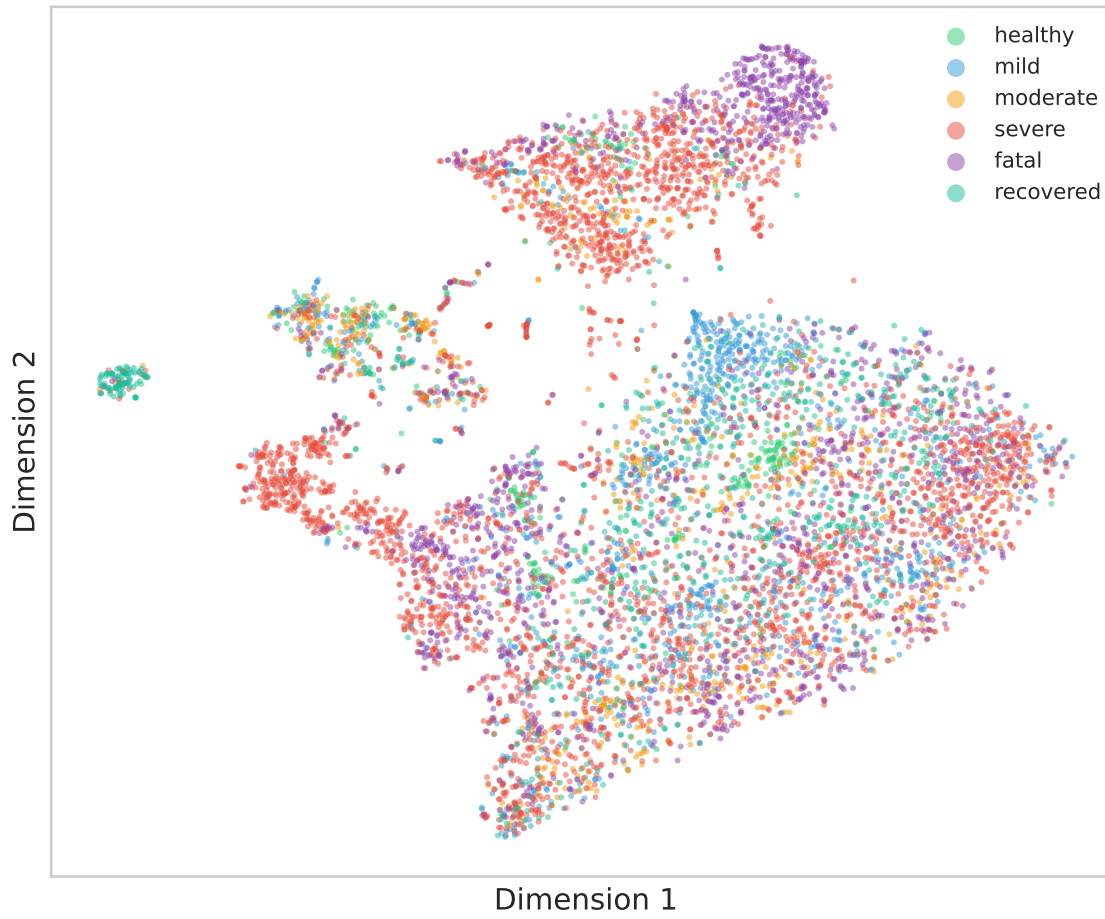
UCE - tSNE
