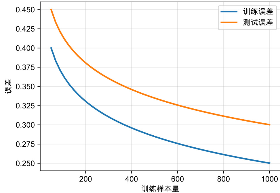
欠拟合 ( 高偏差 )
