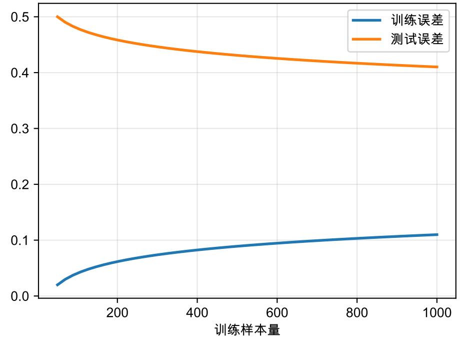
过拟合 ( 高方差 )
