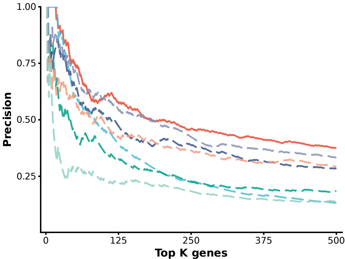
BRCA
