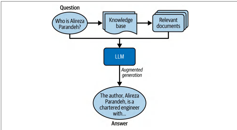
Figure 5-7. RAG
