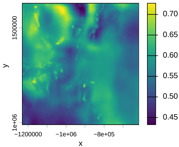
SD, bio1
