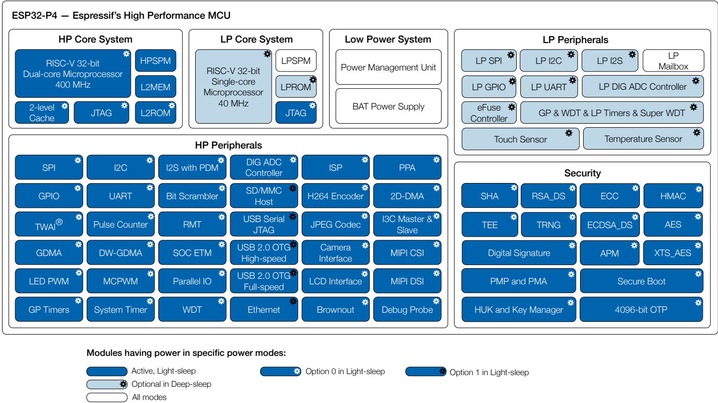
ESP32-P4 功能框图
