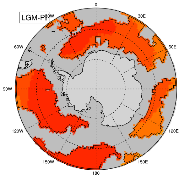
LGM-PI (3900m)
