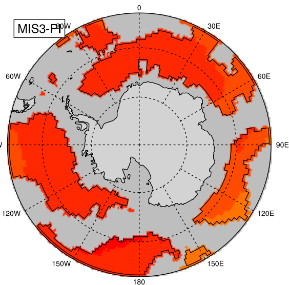
MIS3-PI (3900m)
