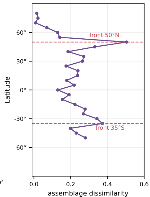
(d) Zonal mean
