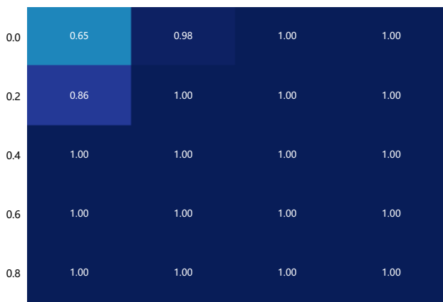
归一化下限×权重联合敏感性 (算术聚合)
