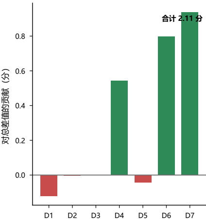
PPO相对A2C的维度贡献
