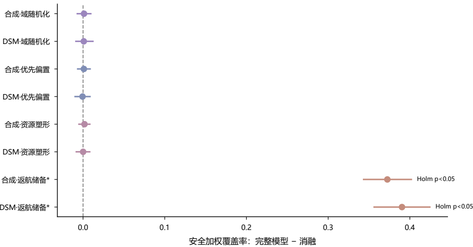
合成与真实DSM的地图级消融效应
