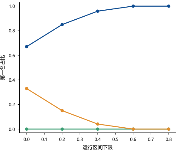
几何聚合 (诊断)
