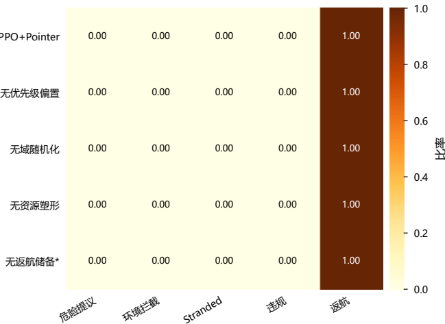
安全行为与失败模式
