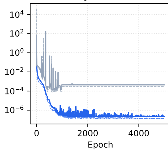
Softsign — 603.8x
