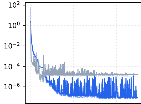
Sigmoid — 54.8x
