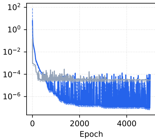
Sin — 459.1x
