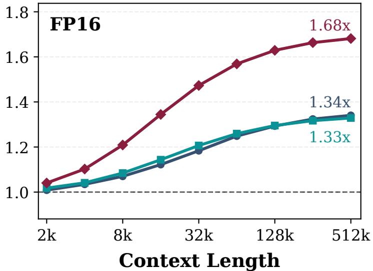
E2E Speedup over FlashAttention
