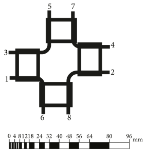
Figura 2 – Topologia de matriz de butler utilizada.
