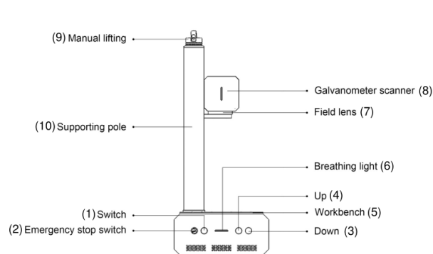
Figura 2: Visão frontal da gravadora
