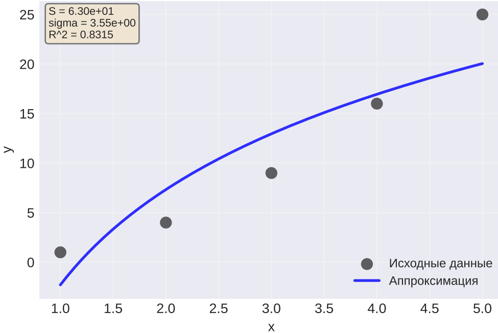
Логарифмическая: f(x) = a \cdot \ln(x) + b
