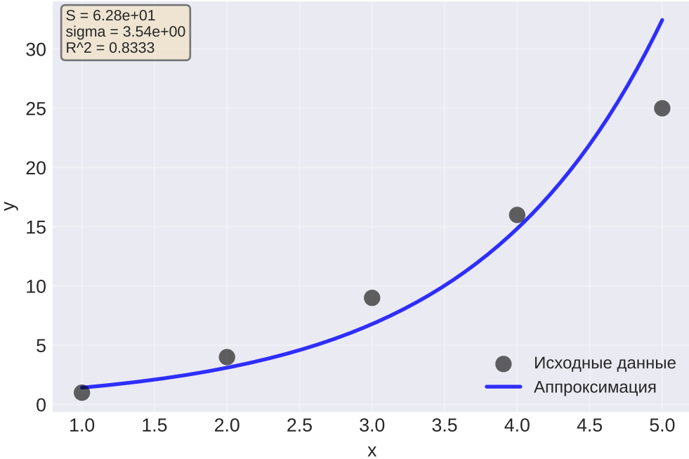
Экспоненциальная: f(x) = a \cdot \exp(b \cdot x)
