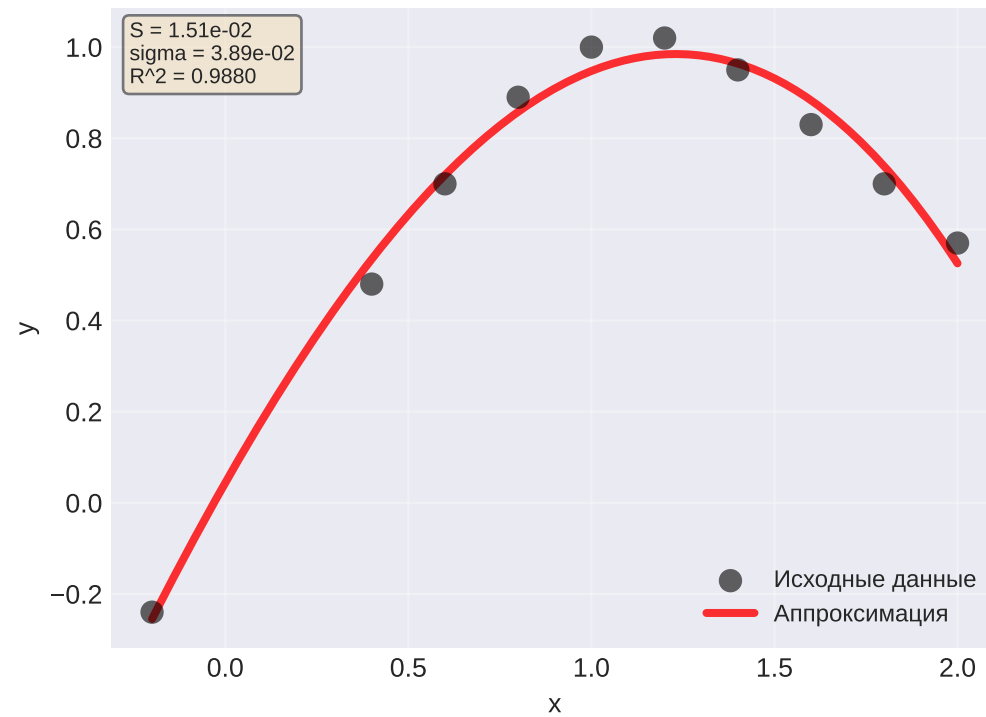
Полином 3: f(x) = a_0 + a_1 \cdot x + a_2 \cdot x^2 + a_3 \cdot x^3 [BEST]
