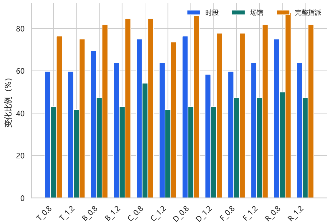
(b) 具体排程替代性
