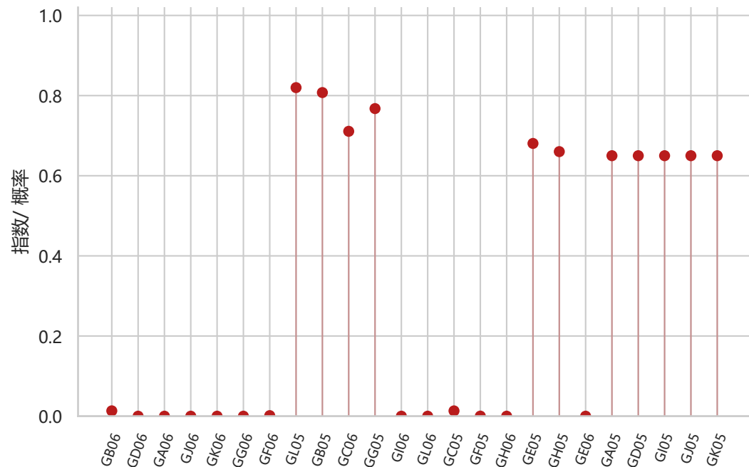
默契风险
