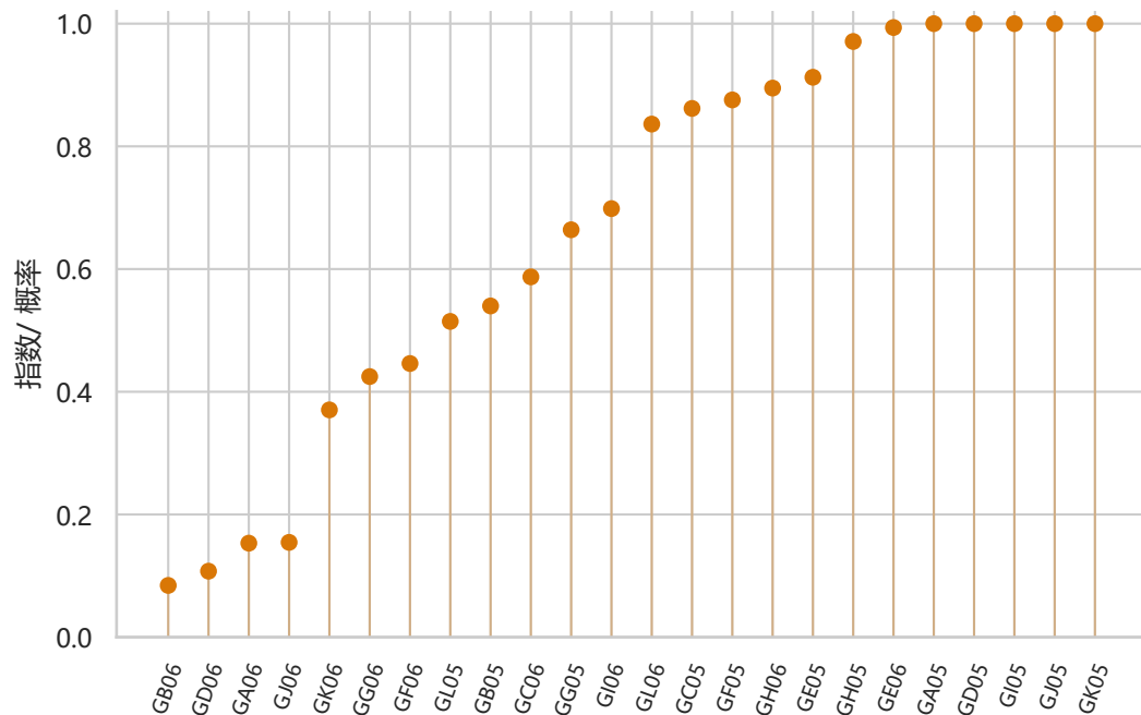
无激励风险
