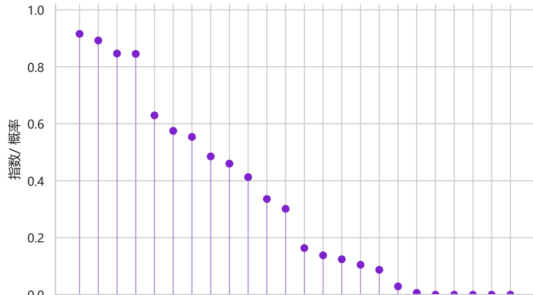
晋级重要性
