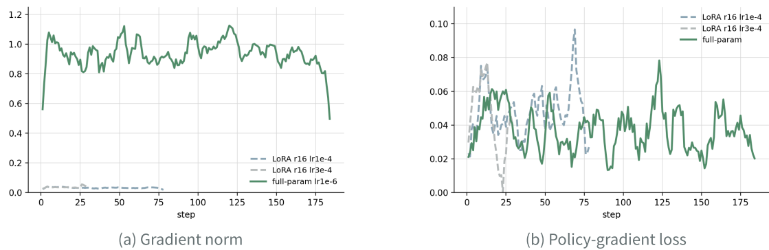
图 B1 · 更新通道诊断。full-param lr=1e-6 保持稳定更新，LoRA (r16) 在 lr=1e-4/3e-4 下有效更新弱一个量级：(a) 梯度范数、(b) 策略梯度损失。
