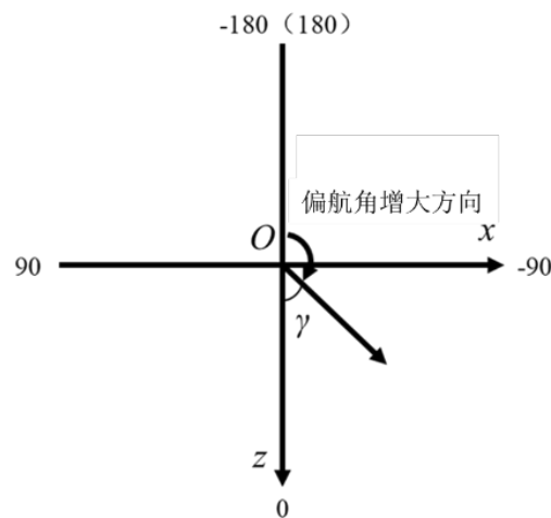
图 2.9 偏航角
