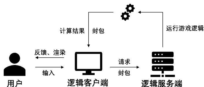
图 1.5 逻辑客户端和逻辑服务端的运行流程
