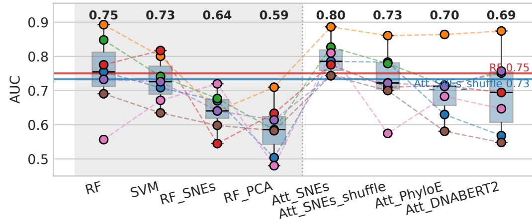
CRC
