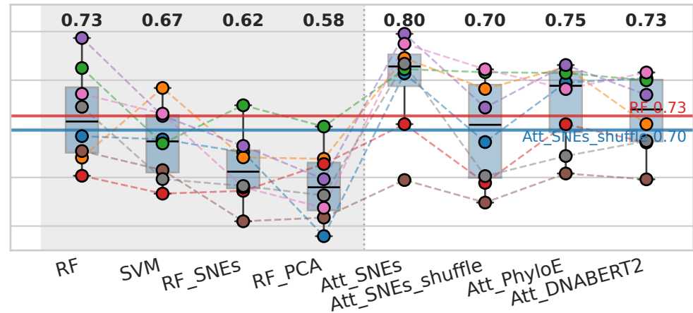
IBD
