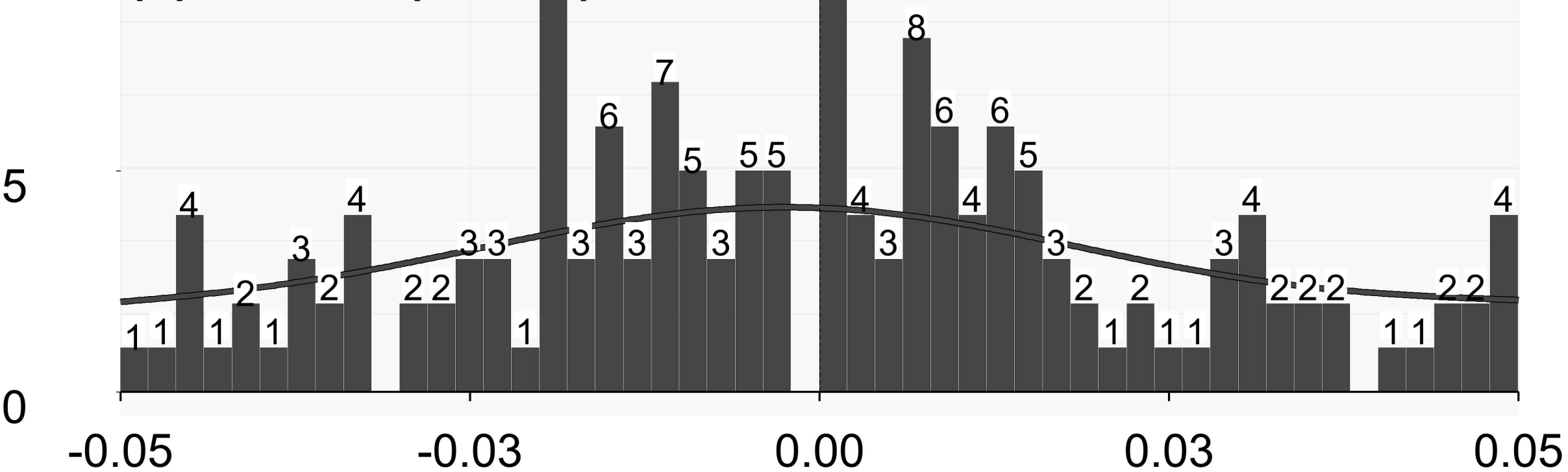
(c) Linear (n=230)
