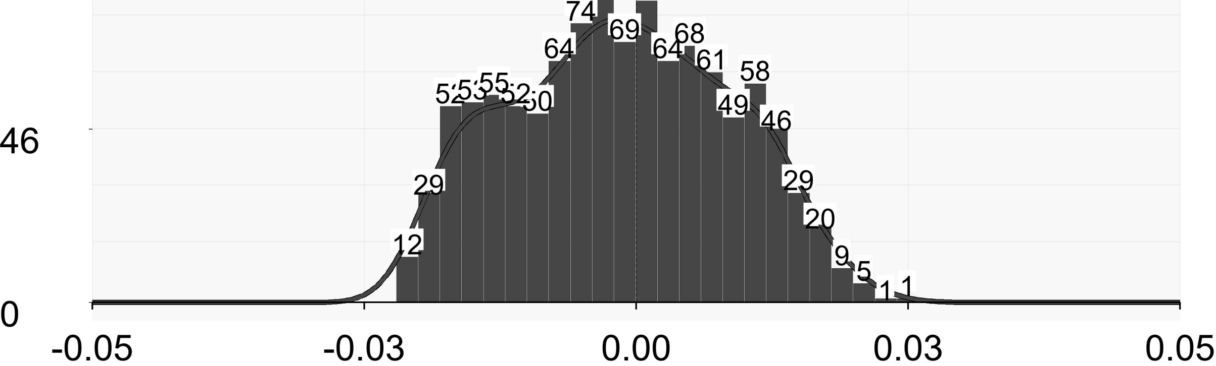
(c) Linear (n=1083)
