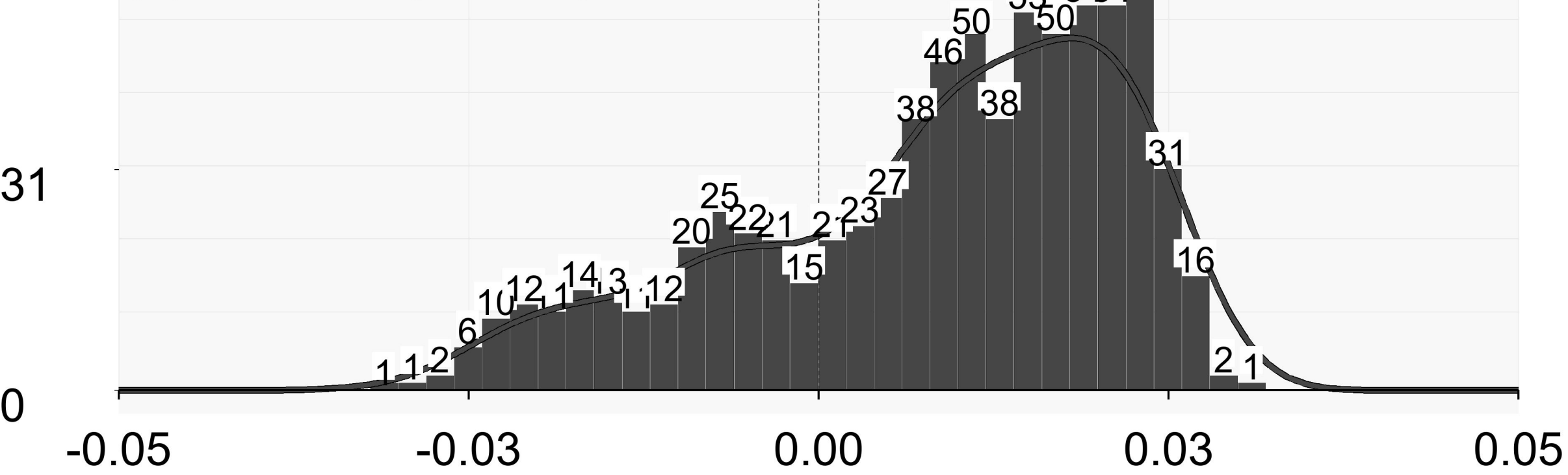
(c) Linear (n=756)
