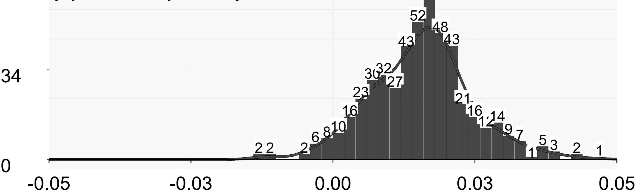
(c) Linear (n=496)
