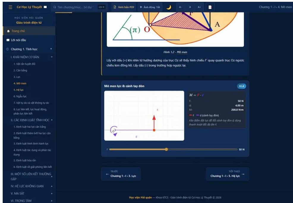
Hình 9. Bước 2–4: O cố định; giữ F = 50 \text{ N} và kéo điểm đặt lực đến d \perp = 4,00 \text{ m} để đọc M = 200 \text{ N}\cdot\text{m} . Nguồn: EV-IMG-07; assets/designs/bao-cao-nghiem-thu-giao-trinh-dien-tu/assets/img-04-mo-men-ch1-1-4-1440x1000.png; SHA-256 bfe78d071e7c712842385f1ba30f9ac046a4a89071c4f9b489b320798e85a57b; thẩm quyền: browser capture bound to presentation evidence; not independent review.
