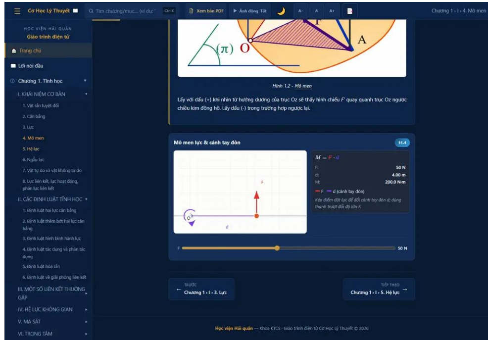
Hình 9. Bước 2–4: O cố định; giữ F = 50 \text{ N} và kéo điểm đặt lực đến d \perp = 4,00 \text{ m} để đọc M = 200 \text{ N}\cdot\text{m} . Nguồn: EV-IMG-07; assets/designs/bao-cau-nghiem-thu-giao-trinh-dien-tu/assets/img-04-mo-men-ch1-1-4-1440x1000.png; SHA-256 bfe78d071e7c712842385f1ba30f9ac046a4a89071c4f9b489b320798e85a57b; thẩm quyền: browser capture bound to presentation evidence; not independent review.
