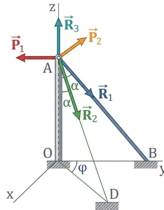
Hệ lực không gian · hình canonical Chương 1
