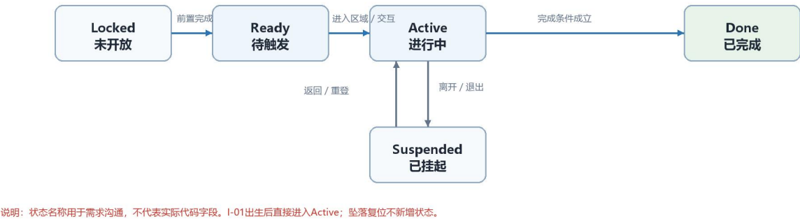
图 3-2 教学步骤状态流转
