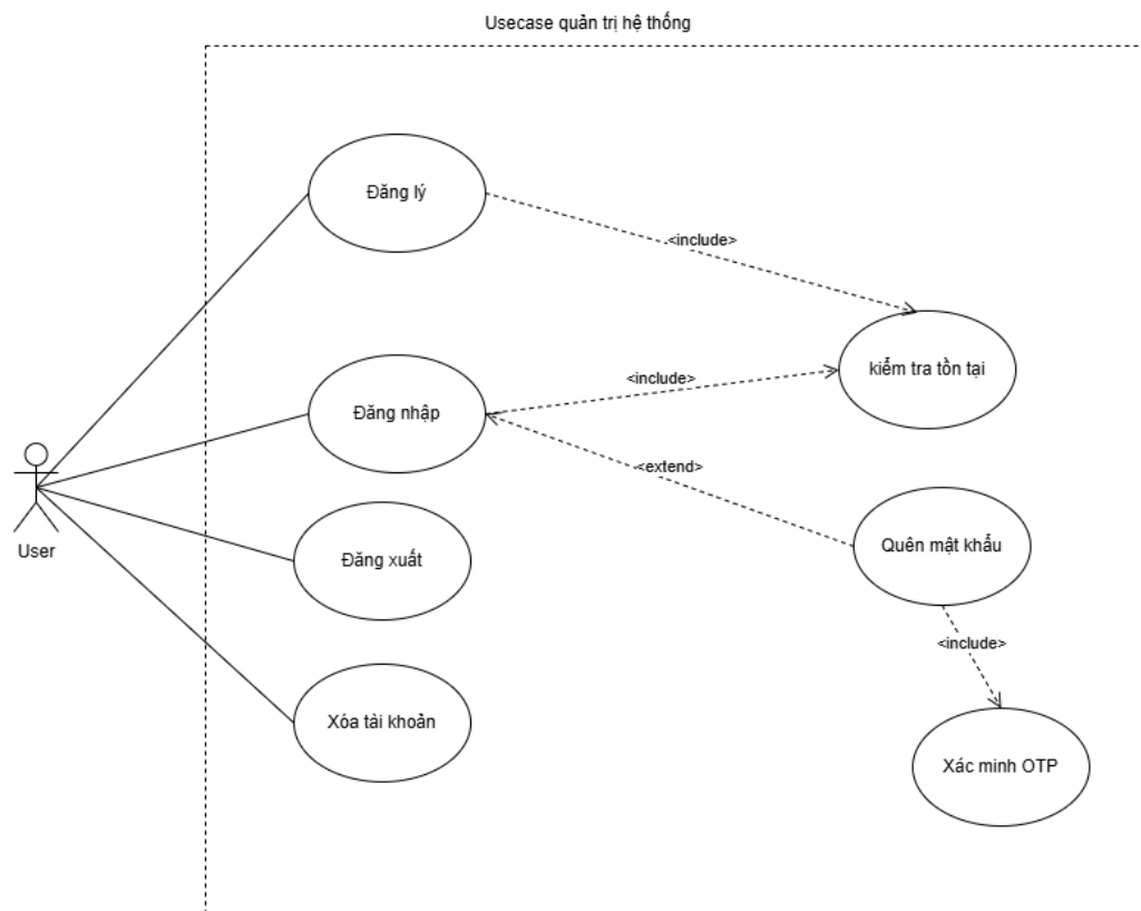
Hình 2.2 Sơ đồ Usecase quản trị hệ thống
