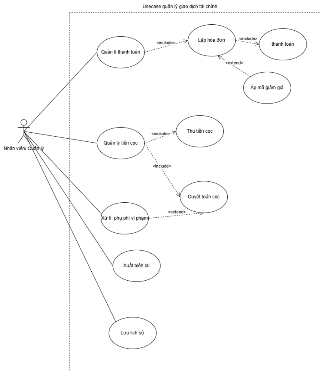
Hình 2.6 Sơ đồ Usecase giao dịch tài chính
