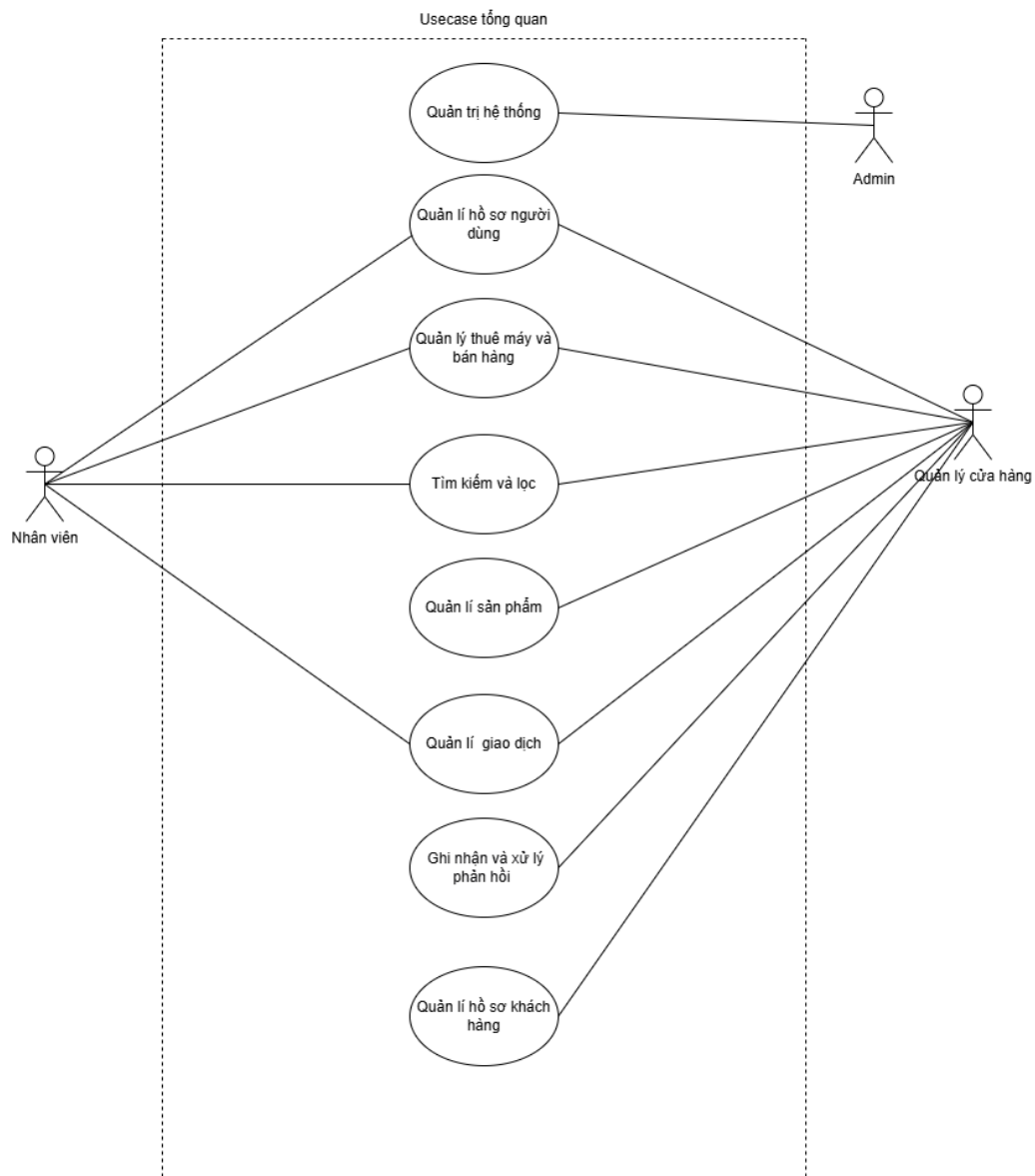
Hình 2.1 Sơ đồ Usecase tổng quan
