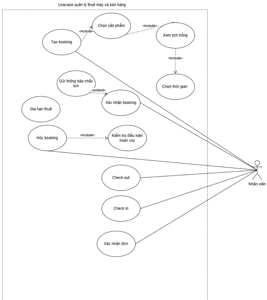
Hình 2.5 Sơ đồ Usecase quản lý thuê máy và bán hàng
