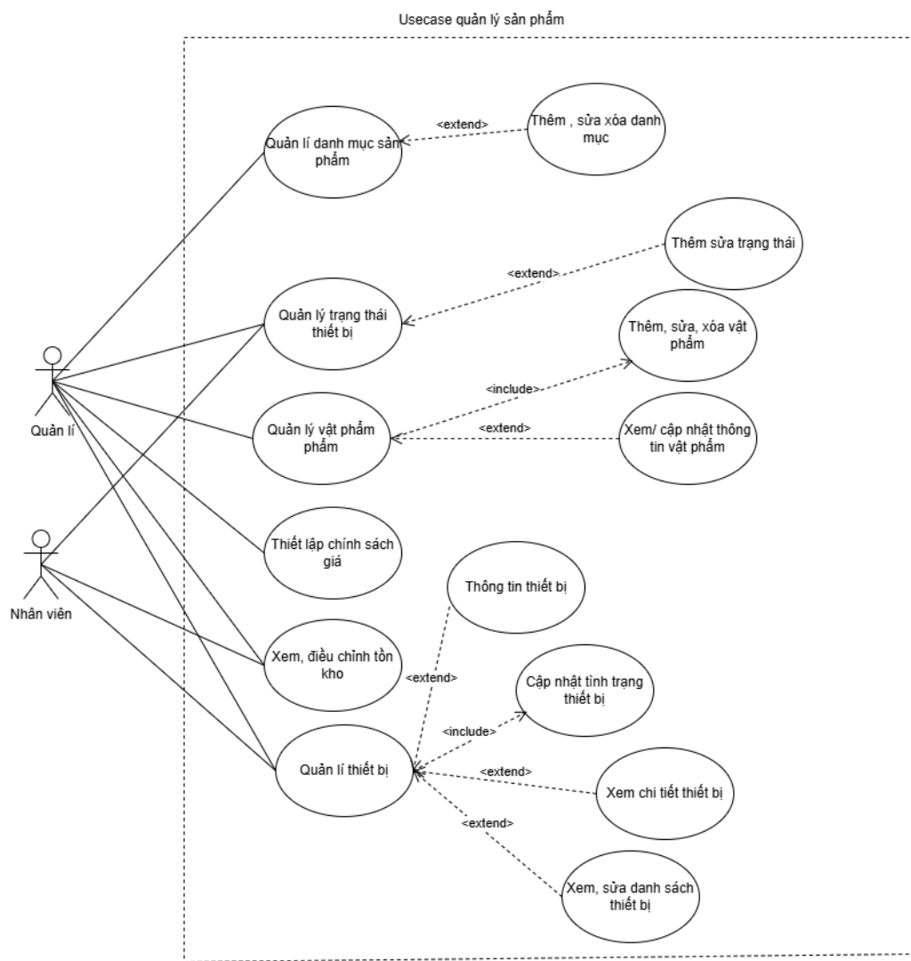
Hình 2.4 Sơ đồ Usecase quản lý sản phẩm
