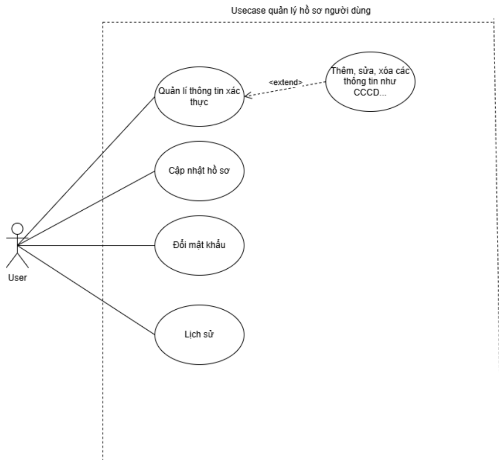
Hình 2.3 Sơ đồ Usecase quản lý hồ sơ người dùng
