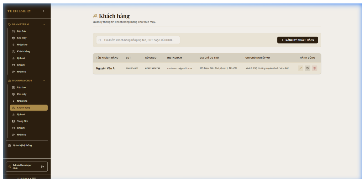
Hình 1.24: Usecase Quản lý khách hàng – Danh sách và tìm kiếm
