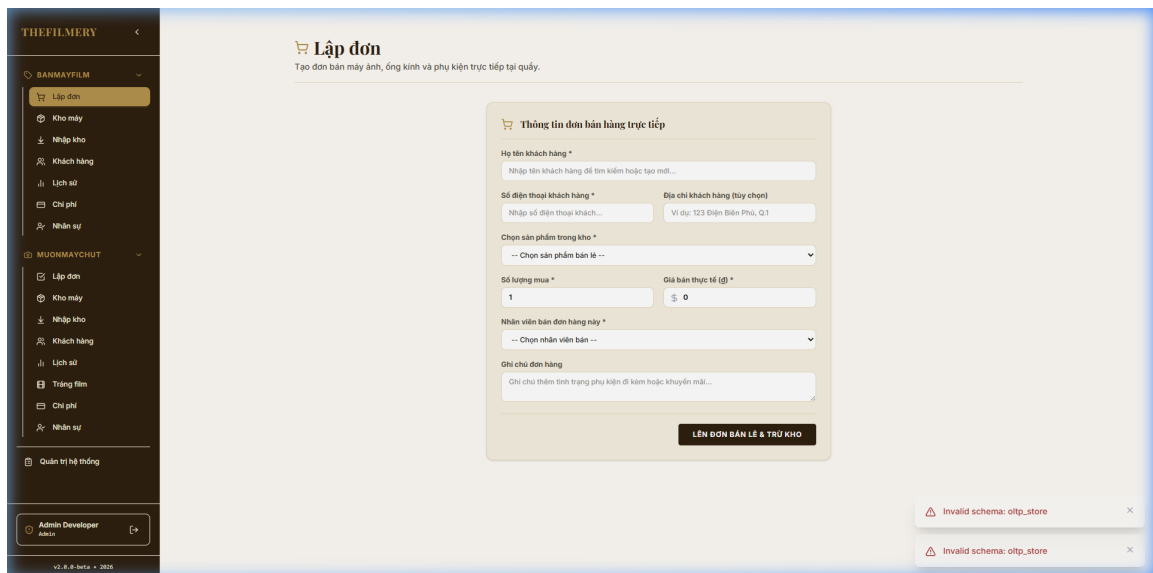
Hình 1.26: Usecase Bán hàng – Giao diện lập đơn bán hàng
