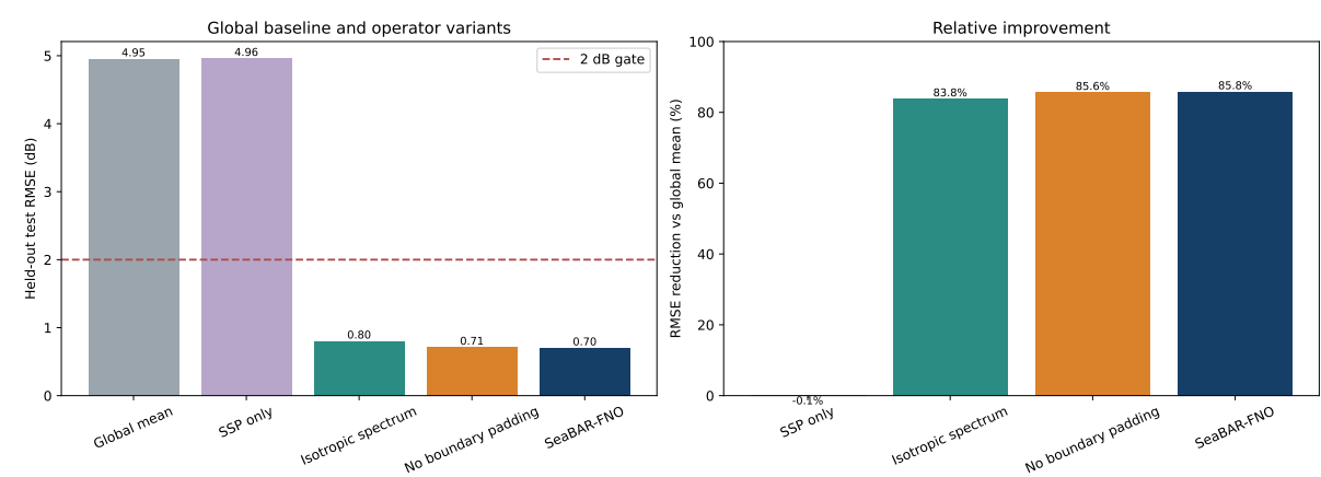
图 5: 全局均值场、仅 SSP 变体和三个含地形算子变体的测试 RMSE，以及相对全局均值场的降幅。
