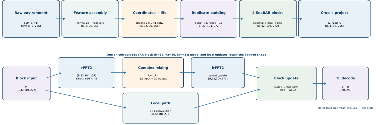
图 4: 最终 SeaBAR-FNO 的端到端张量维度，以及单个各向异性 Fourier 模块内部的谱路径、局部路径和 dB 解码。B 表示 batch size。
