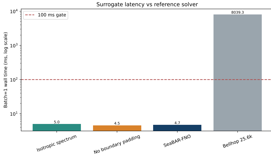
图 10: 三个含地形 FNO 变体的 batch=1 P95 时延与 25,600 射线 Bellhop 单场中位耗时。纵轴采用对数尺度。
