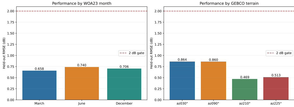
图 6: SeaBAR-FNO 在 WOA23 3/6/12 月和四类 GEBCO 地形上的密封测试 RMSE；所有子组均通过 2 dB 门槛。
