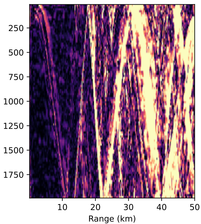
Absolute error
