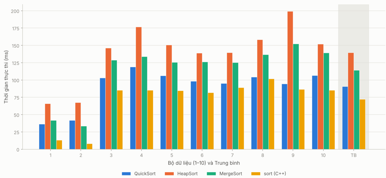
So sánh thời gian thực thi của QuickSort, HeapSort, MergeSort và std::sort (mỗi dãy ~1.000.000 số thực)
