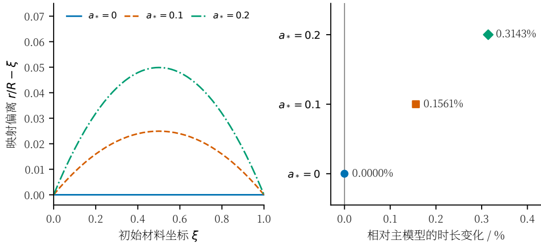
图 17 内部映射正向扰动的代表性结果；左图取 t = 51.0775 \text{ h} ，右图为未标定情景的计算结果，双侧扰动数值见正文
