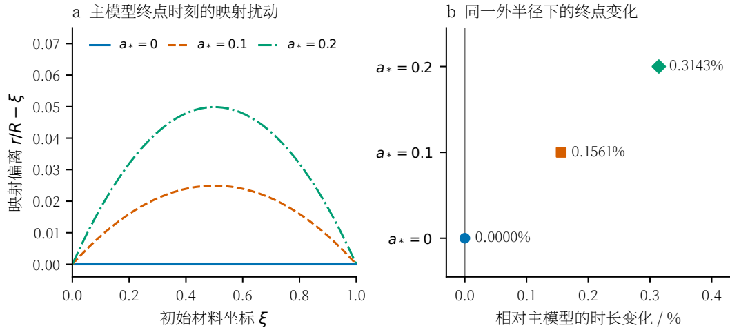
图 15 内部映射扰动及其对干燥时长的确定性影响; 左图取 t = 51.0775 h, 右图为未标定情景的计算结果
