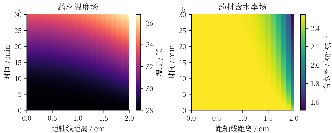
图 2 问题一热湿径向场
