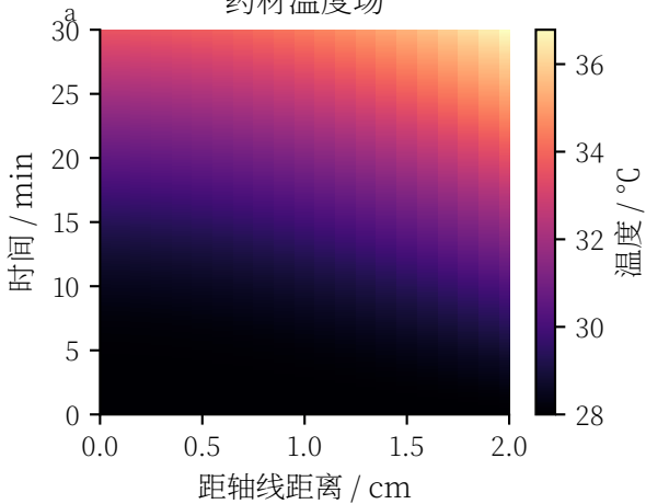
药材温度场
