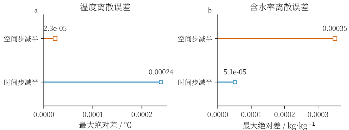
图 3 问题一时间步与空间步加密误差
