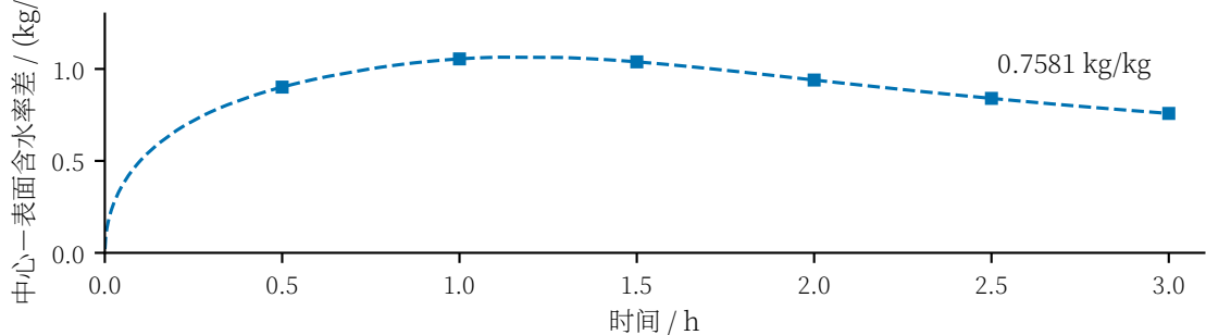
b 含水率差在 3 h 时仍然存在
