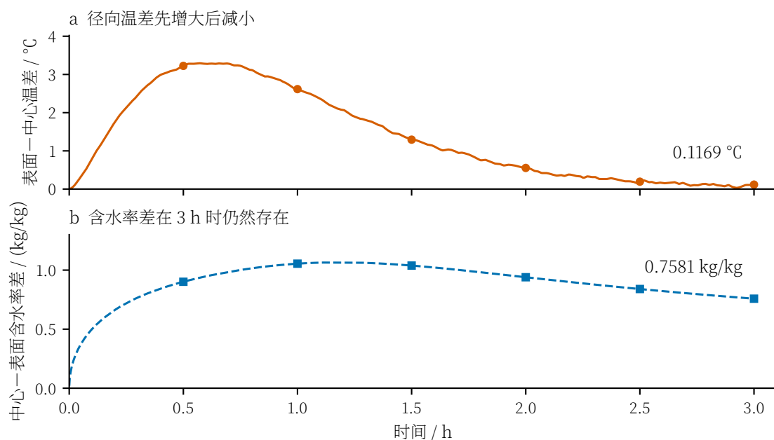
图 7 问题二中心与表面之间的温差和含水率差；标记对应每隔半小时的报告时刻
