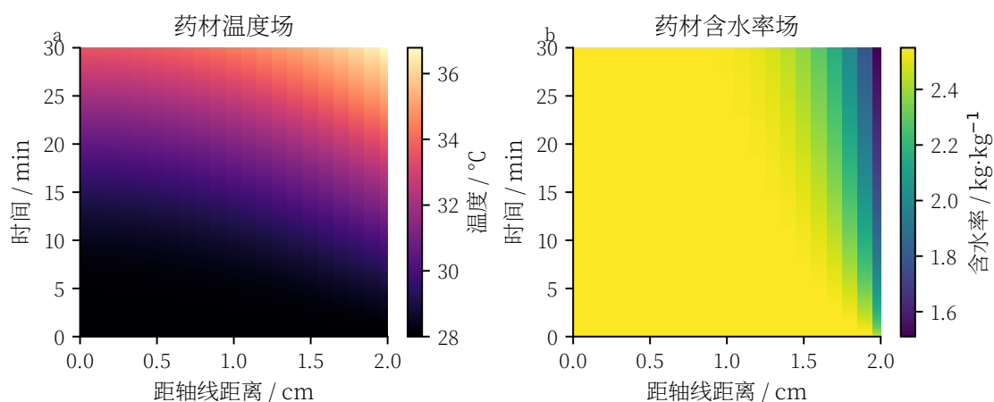
图2 问题一温度与干基含水率径向场
