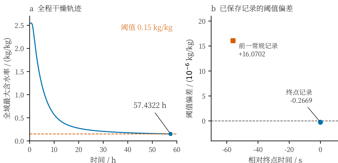
图 9 问题三全域最大含水率及终点阈值偏差；右图为相隔 56 s 的两条已保存记录，首次时刻由 1 s 步长检测确定
