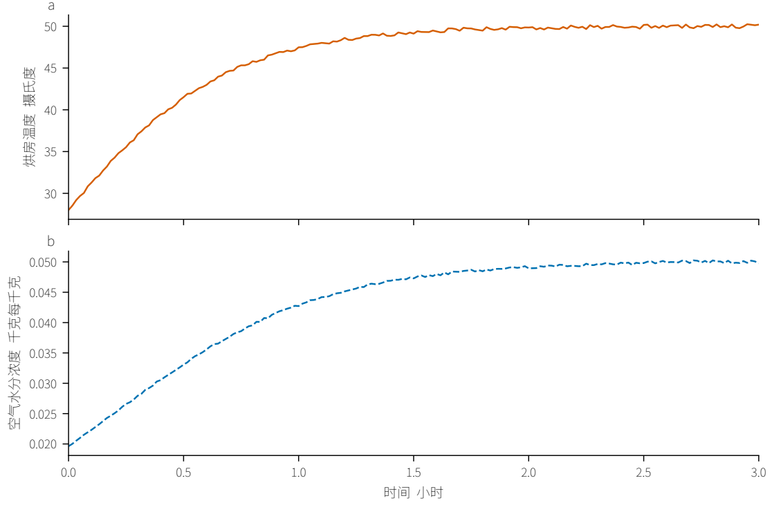
图 4 问题二前三小时的空气边界
