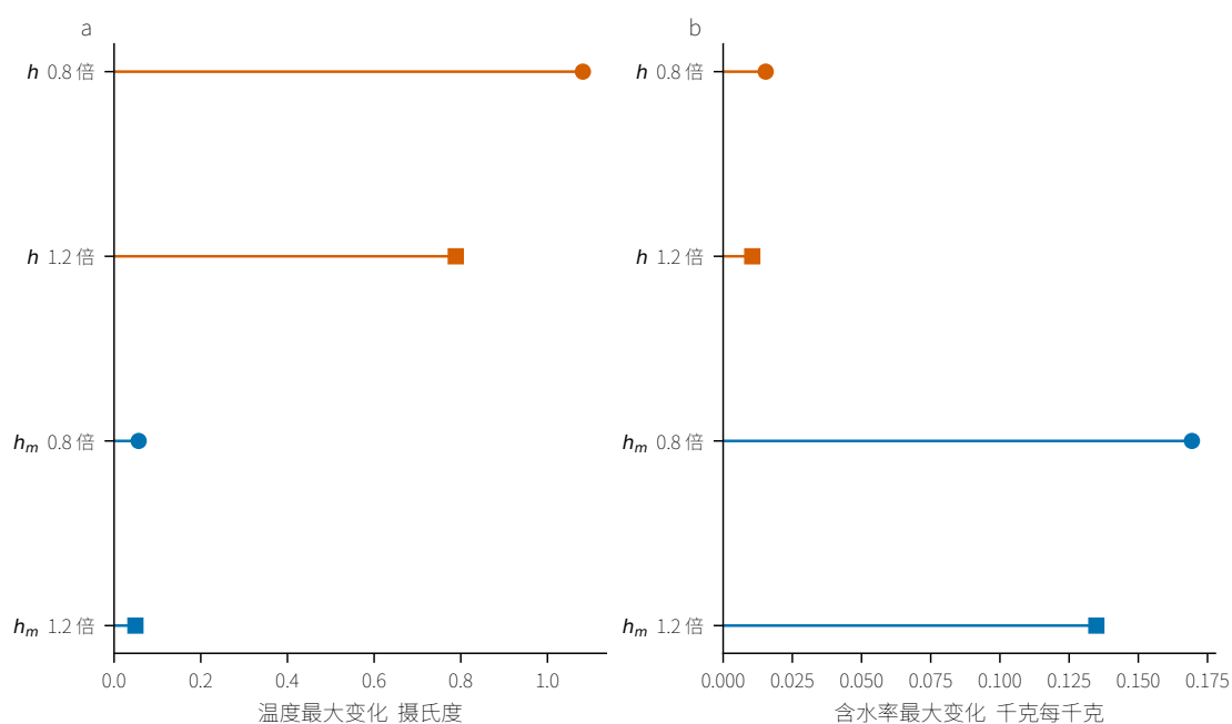
图 8 问题二边界参数在三十个报告点上的确定性灵敏度
