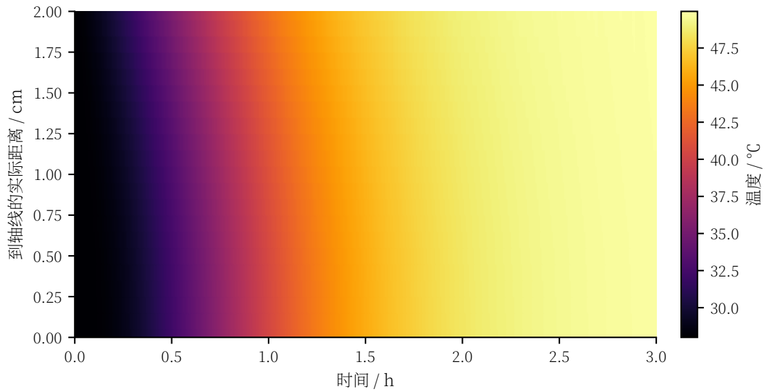
图 5 问题二前三小时的径向温度场
