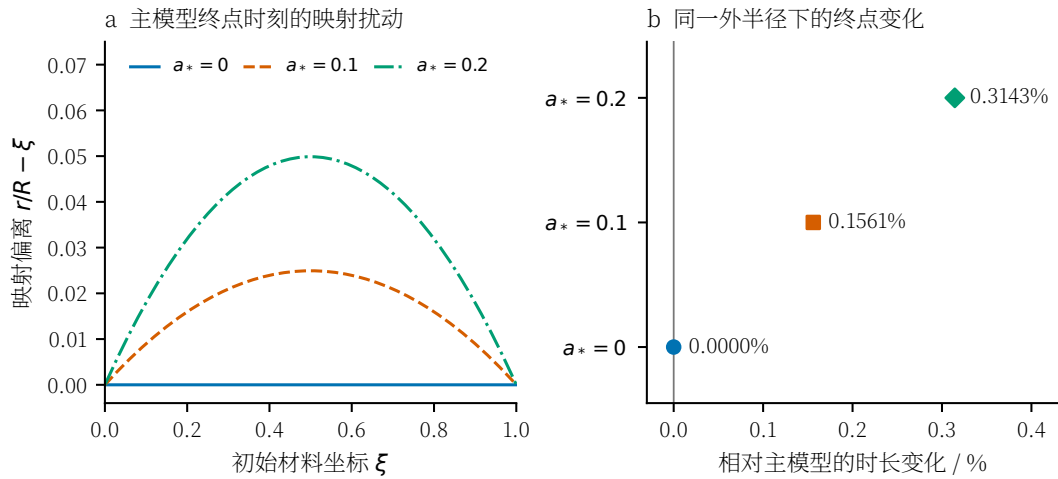
图 15 内部映射正向扰动的代表性结果；左图取 t = 51.0775 h，右图为未标定情景的计算结果，双侧扰动数值见正文
