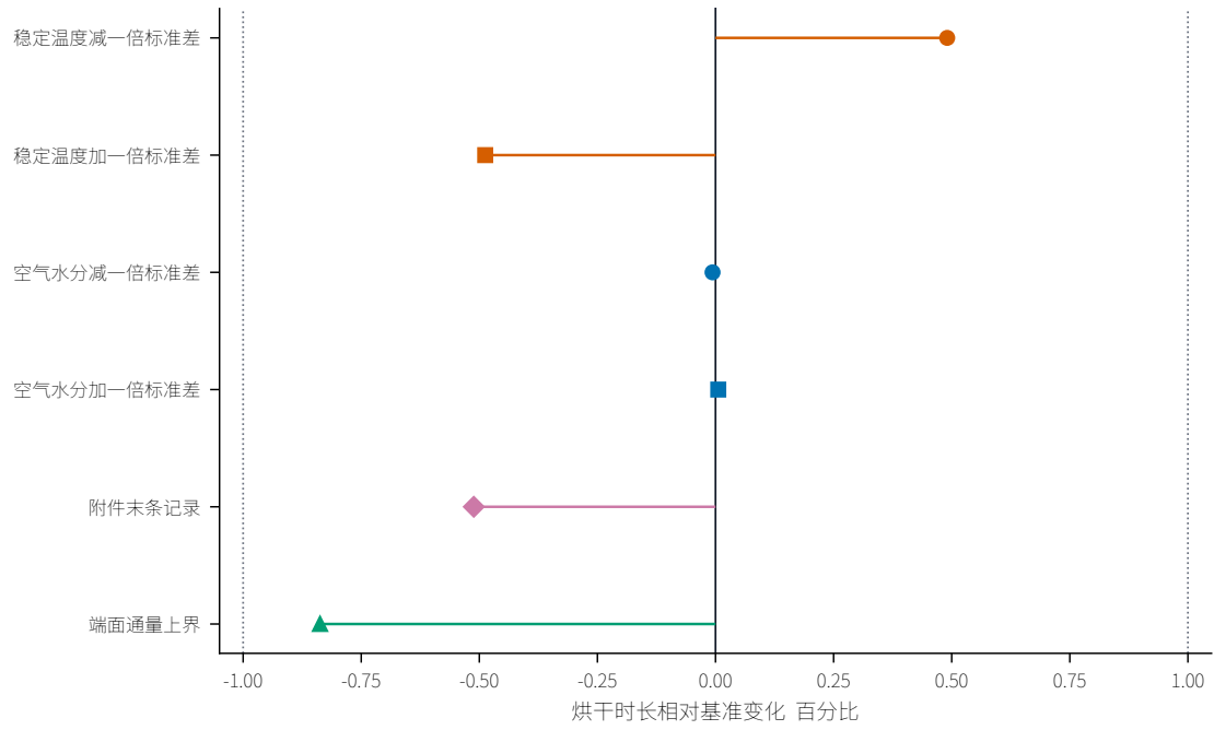
图 11 问题三长期空气边界与集总系数扰动情景
