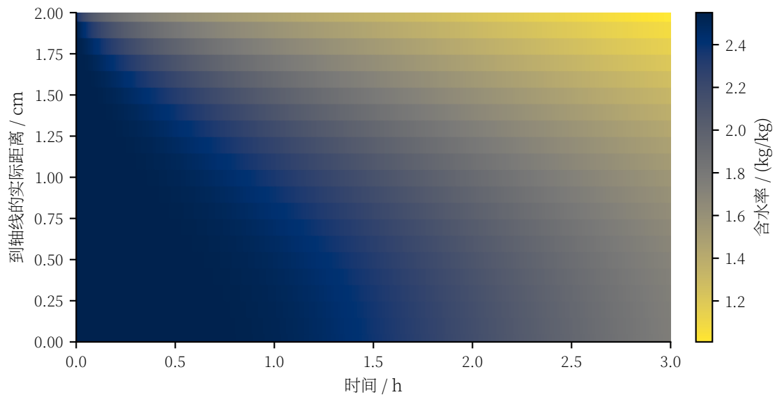
图 6 问题二前三小时的径向干基含水率场
