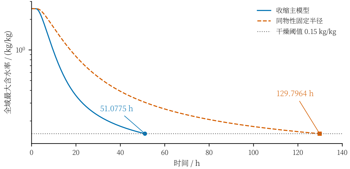
图 14 同附录四物性下收缩模型与固定半径对照的阈值跨越；纵轴采用对数刻度
