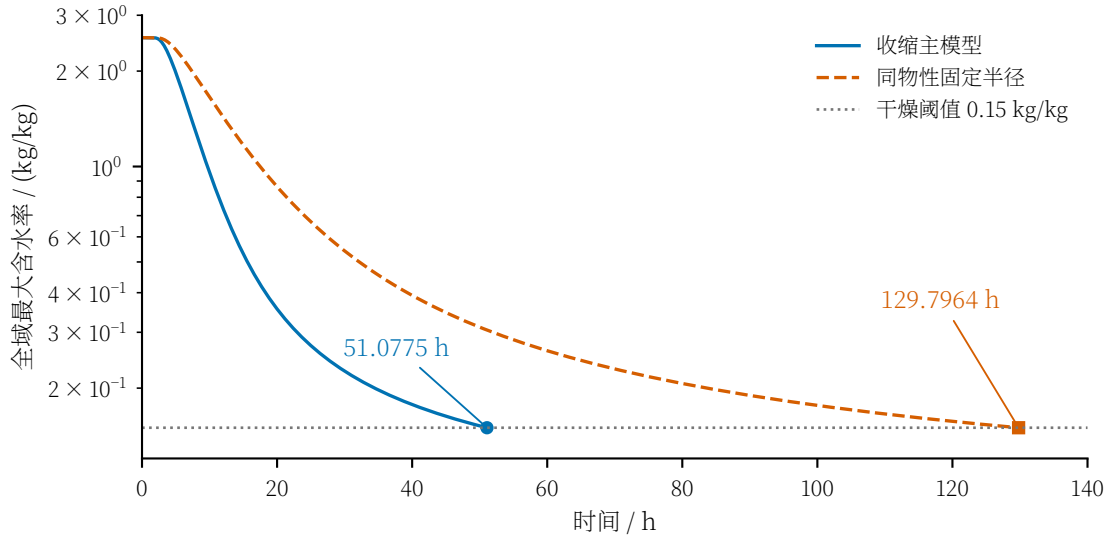
图 14 同附录四物性下收缩模型与固定半径对照的阈值跨越；纵轴采用对数刻度
