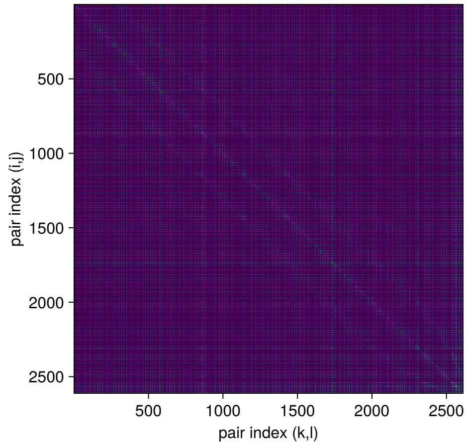
\log_{10}|V_{ij,kl}| (eV), 2611×2611
