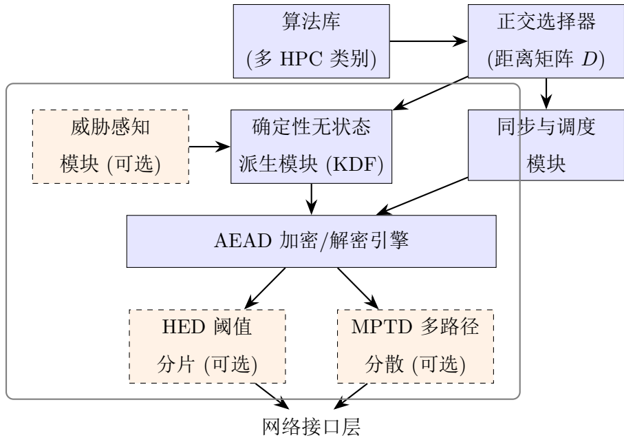
图 1: DMHP 节点总体架构图
