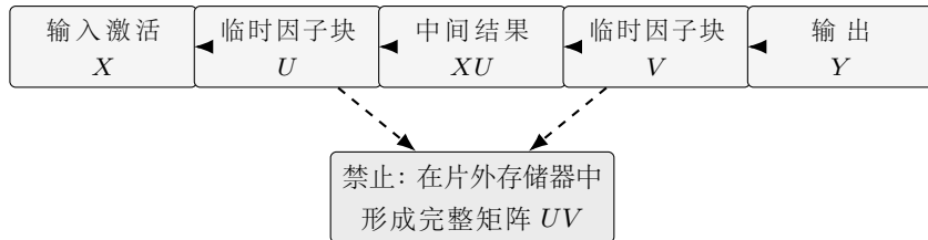
图 4 基于结合律的矩阵执行与禁止片外物化示意图
