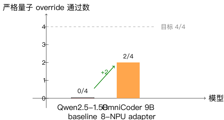
图 12: 严格量子 holdout 上的 override-only 成绩对比。两根柱子对应的 run 共享相同的 4 个 task、prompt_version=v2、prompt_style=repair_focused、include_reference_candidate=false 与 token_budget_preset=quantum_heavy；OmniCoder base 9B 的第三根柱子当前仍缺失，因为 2026-04-10 fresh ai2 回评先卡在模型快照恢复。
