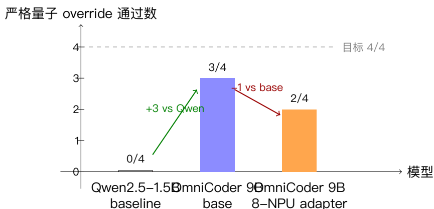
图 12: 严格量子 holdout override 成绩对比。三组 run 共享相同评测协议。
