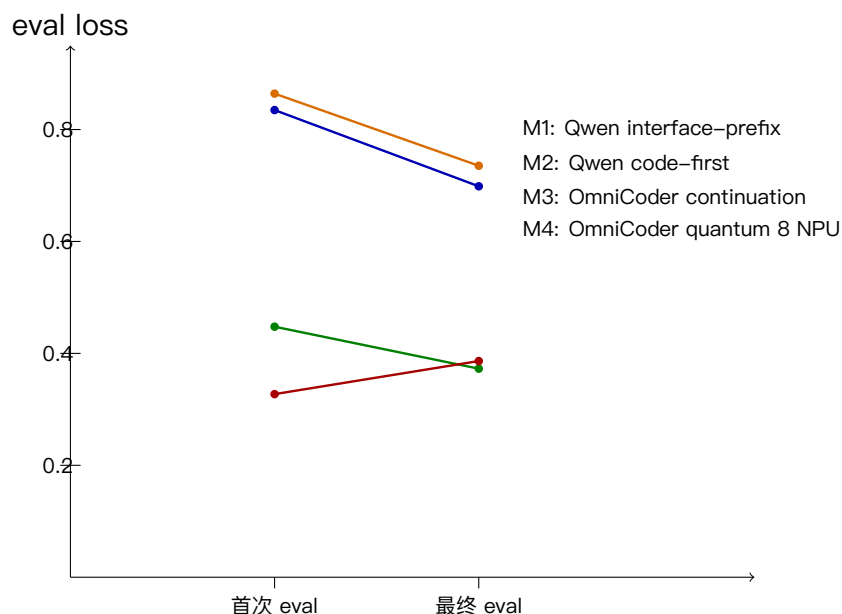
图 9: 四组训练工件在首次 eval 点与最终 eval 点的变化。
